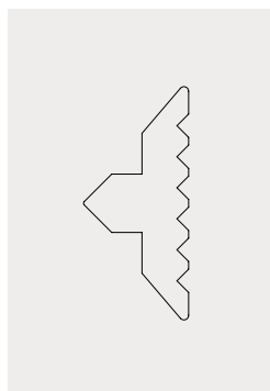
justo FLIPP Kontaktprofil EPDM-Dichtung grau justo FLIPP Contact Profile EPDM grey sealing feste Länge | fix length für 8/10/12 mm Glas | for 8/10/12 mm glass Art. 36801700135 200 m für 8/10/12 mm Glas | for 8/10/12 mm glass Art. 36801700138
