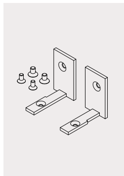
justo FLIPP Verbinder zwischen Zargenprofil und Wandanschlussprofil (Set) justo FLIPP Connector between frame and WCP (set) Art. 36800800125
