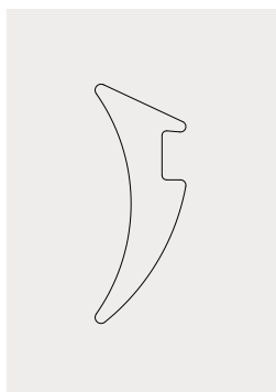
justo FLIPP Glas-Keilprofil EPDM-Dichtung grau justo FLIPP Glass wedge profile EPDM grey sealing feste Länge | fix length für 8 mm Glas | for 8 mm glass Art. 36801500135 für 10/12 mm Glas | for 10/12 mm glass Art. 36801600135 200 m für 8 mm Glas | for 8 mm glass Art. 36801500138 für 10/12 mm Glas | for 10/12 mm glass Art. 36801600138
